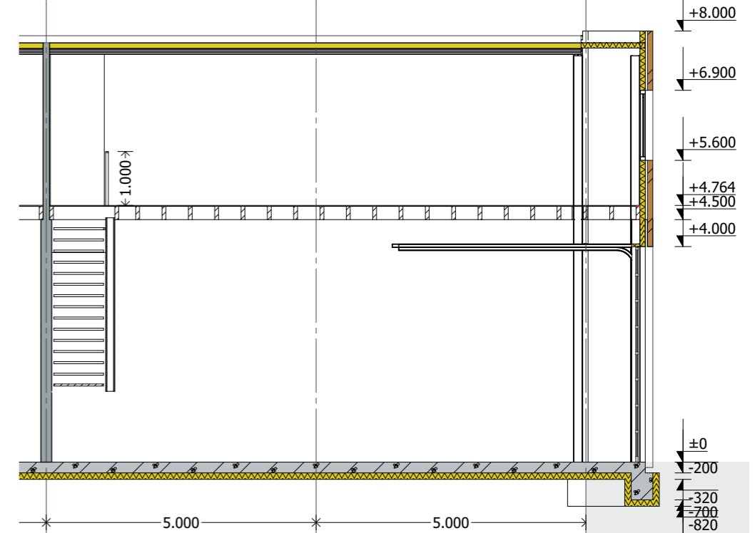
Doorsnede B-B
