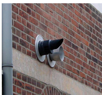
Individuele gevelaansluiting
