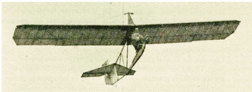
De voorzitter van de zweefvliegclub "Soesterberg" in zijn Zöglin vliegtuig (Bron Utrechts Nieuwsblad d.d. 17-07-1933)
