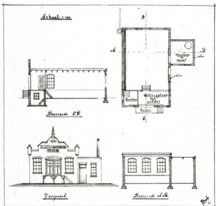
De bouwtekening uit 1907 van het eerste gebouw waarin de zuivelfabriek was gevestigd. We herkennen de gevel van de foto, waarmee het bewijs is geleverd dat de foto inderdaad van de zuivelfabriek op de Middelwijkstraat is.
