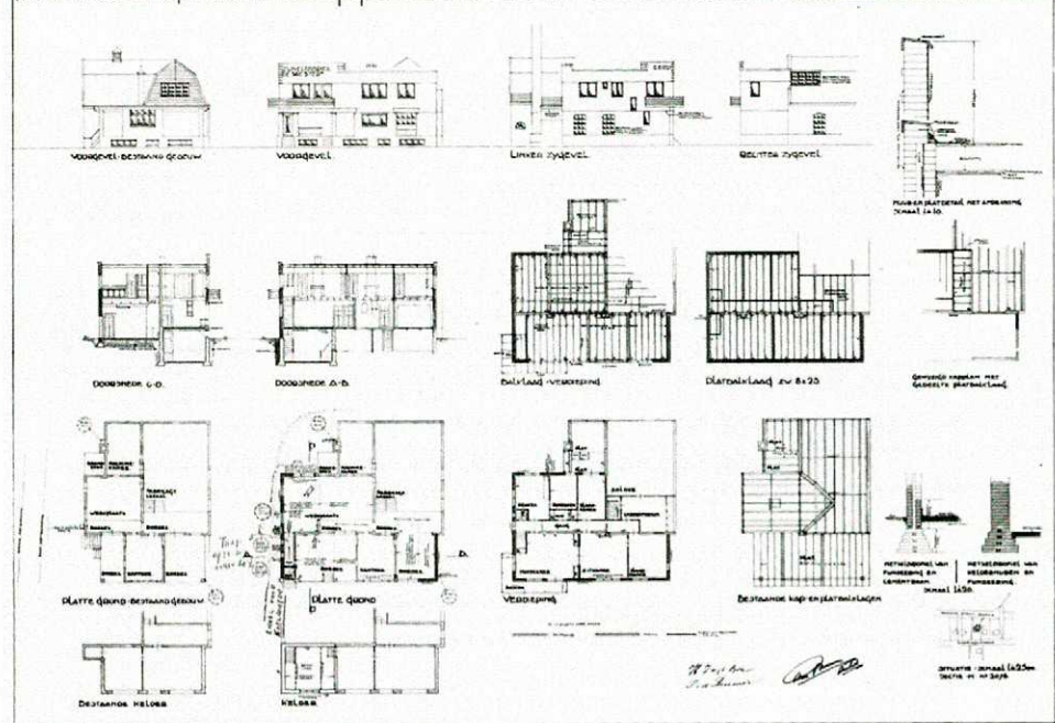
Bouwtekening voor de verbouwing in 1933.
