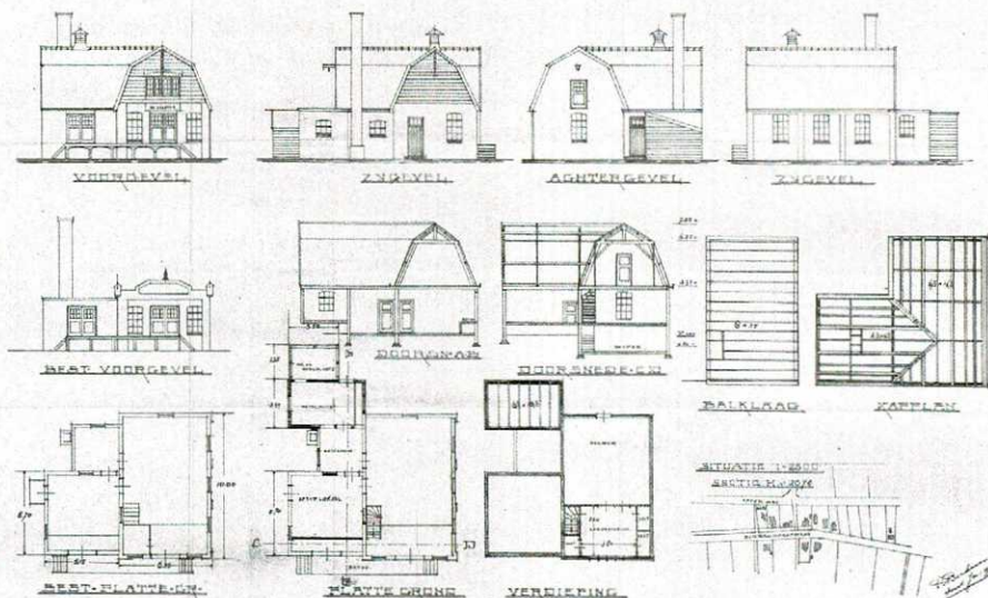
Bouwtekening van het bedrijf uit 1921; de bouw van een extra laag en het mansardedak.
