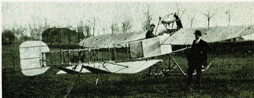
Het door Josephus Jitta in Soesterberg gebouwde toestel, een eendekker uit 1912, voorzien van een 35 pk. Anzani-motor.
