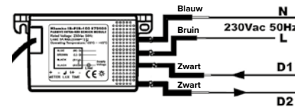
Fig. 3: Aansluitschema
