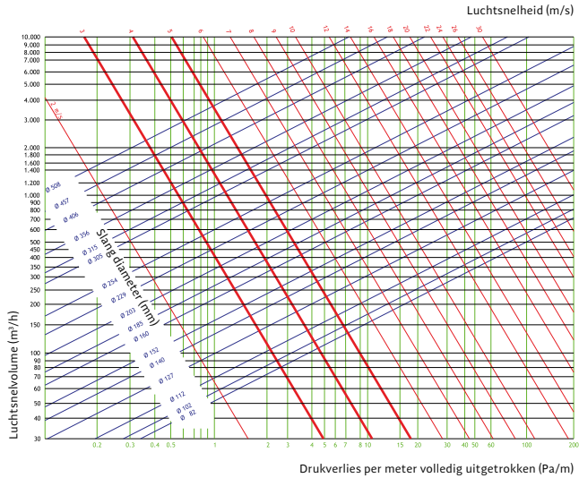
Drukverlies diagram FORTEFLEX
