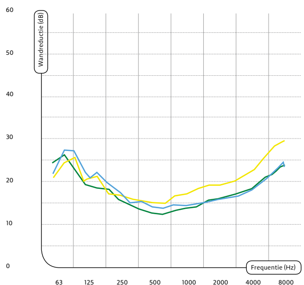
Wandreductie AM2 ISO AKS
