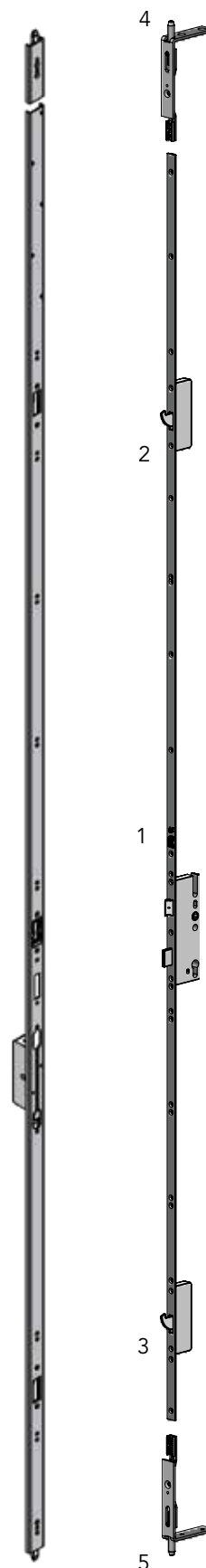
contra-espagnolet vijf sluitpunten
