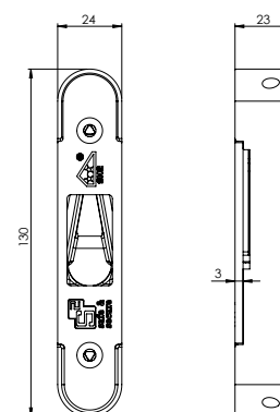
flexi haaksluitkom reno
