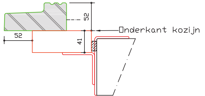
Holonite voor buitendraaiende deur
