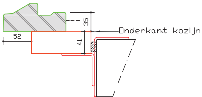
Holonite voor binnendraaiende deur
